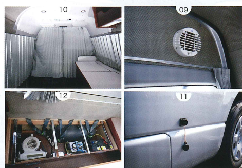
9. リアゲートの上部に設置されている換気口。ゲートの内部を通してボディ下部に排気される。10. フロントシート後ろの間仕切り付き遮光カーテンは標準で装備。ぐるりと全方位遮光できるので、完全にプライバシーを守ることができる。11. 外部電源も標準装備。長期のクルマ旅にありがたい。12. 右側シート下収納庫にはリアヒーターやサブバッテリー等が収納されている。
